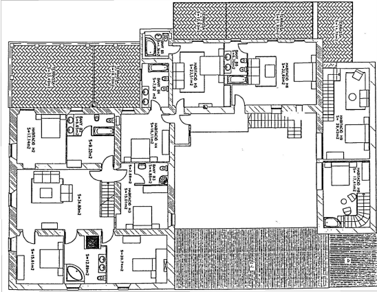
PLANTA PRIMERA
