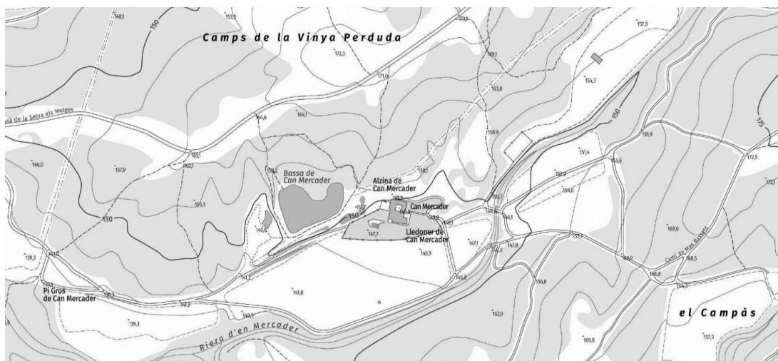
TOPOGRAFIA DE CAN MERCADER SEGONS QUEDA RECOLLIT EN L'INSTITUT CARTOGRAFIC I GEOLOGIC DE CATALUNYA (ICGC) TOPOGRAFIA DE CAN MERCADER RECOGIDA EN EL INSTITUTO CARTOGRAFICO Y GEOLOGICO DE CATALUNA (ICGC)
